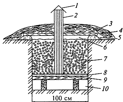
Рис. 4.16. Зимняя непромерзающая траншея:
