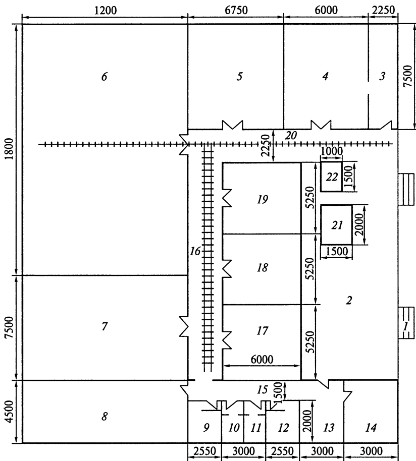
Рис. 6.1. Схема холодильного комплекса по приемке, обработке и хранению посадочного материала:
